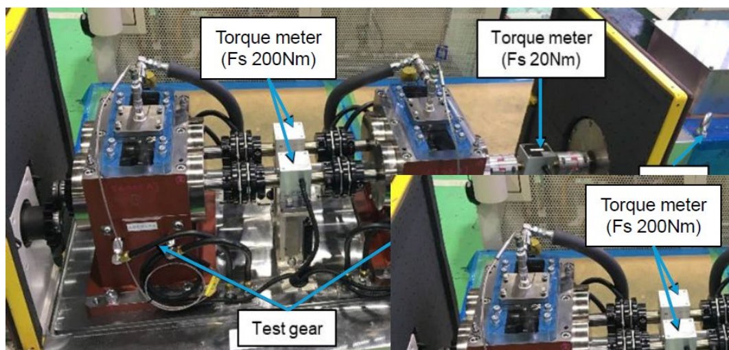
図 1 動力循環式歯車試験機
