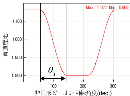
図 38.12 不等速回転角 ( \theta_q )，(角度速比グラフ)
