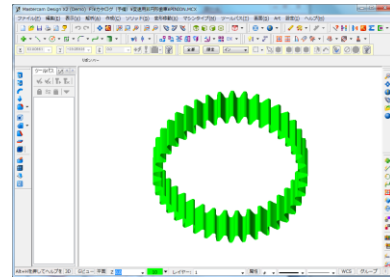
図 38.24 非円形歯車の CAD 作図例 (3D-IGES)
