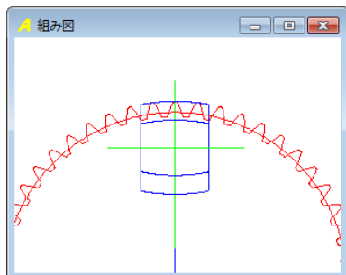
図 39.16 組み図 (ホブと内歯車)
