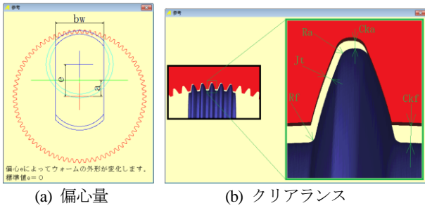
図 39.5 内歯-樽形ウォームの機能
