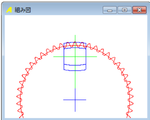
図 39.7 組図 (ウォームと内歯車)
