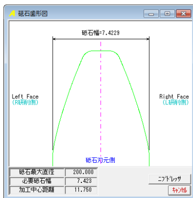
図 16.22 砥石歯形
