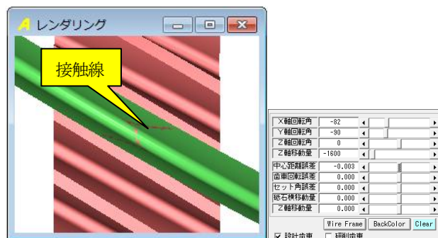
設計歯車と砥石のかみ合い
