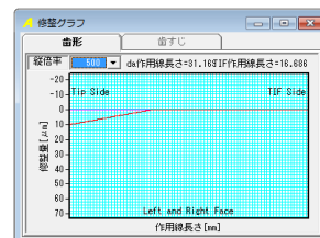
図 16.5 歯形修整グラフ
