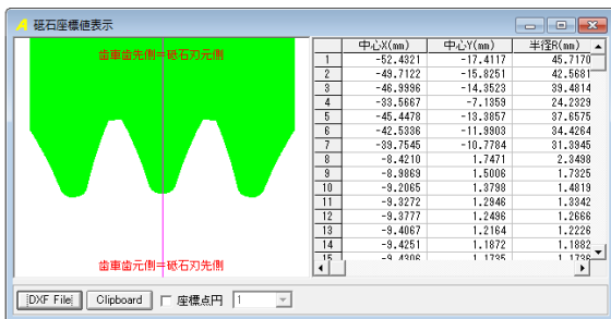
図 16.17 砥石座標（複溝）
