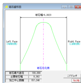
図 16.11 砥石歯形
