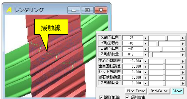
図 16.18 歯形レンダリング（複溝）
