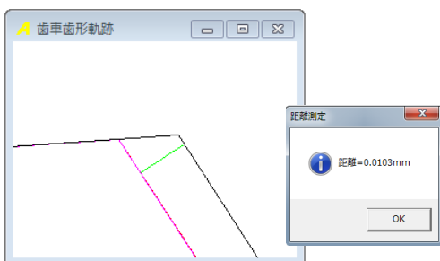
図 16.10 研削歯形と無修整歯形 (距離測定)
