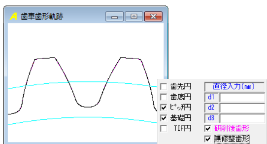
図 16.9 歯車歯形
