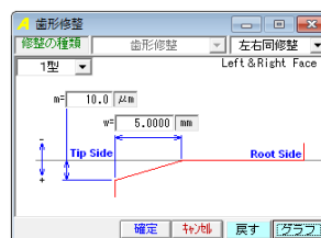
図 16.4 歯形修整 (1 型)
