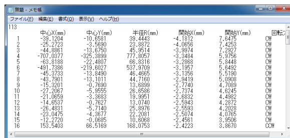
図 16.14 砥石座標
