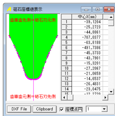
図 16.13 砥石座標
