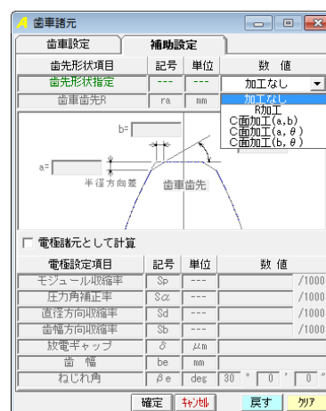
図 16.3 補助設定
