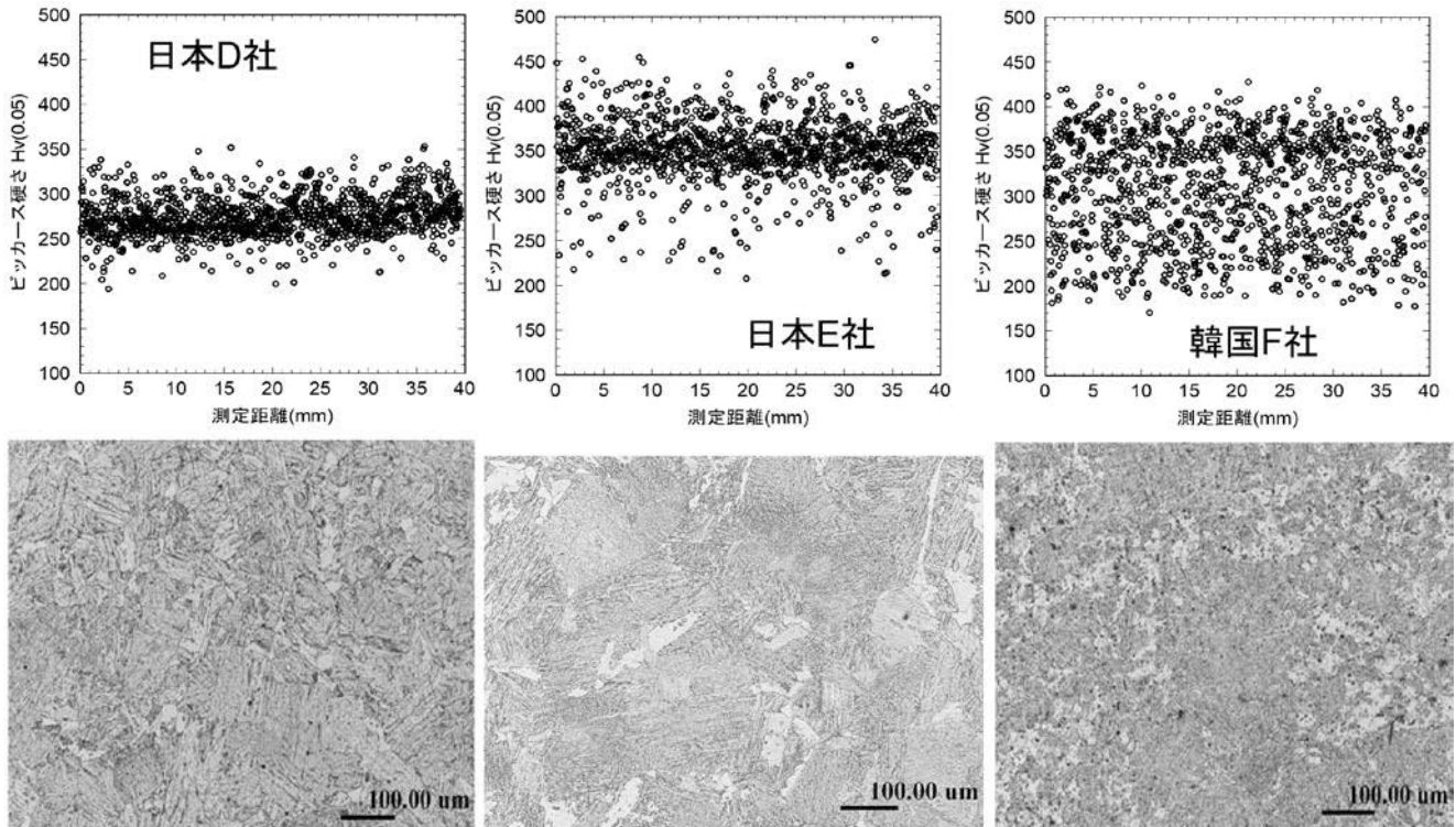
0.17 節「硬さのラツキと鋼材品質」の中の一例：18CrNiMo7-6 材のメーカー別の品質差
